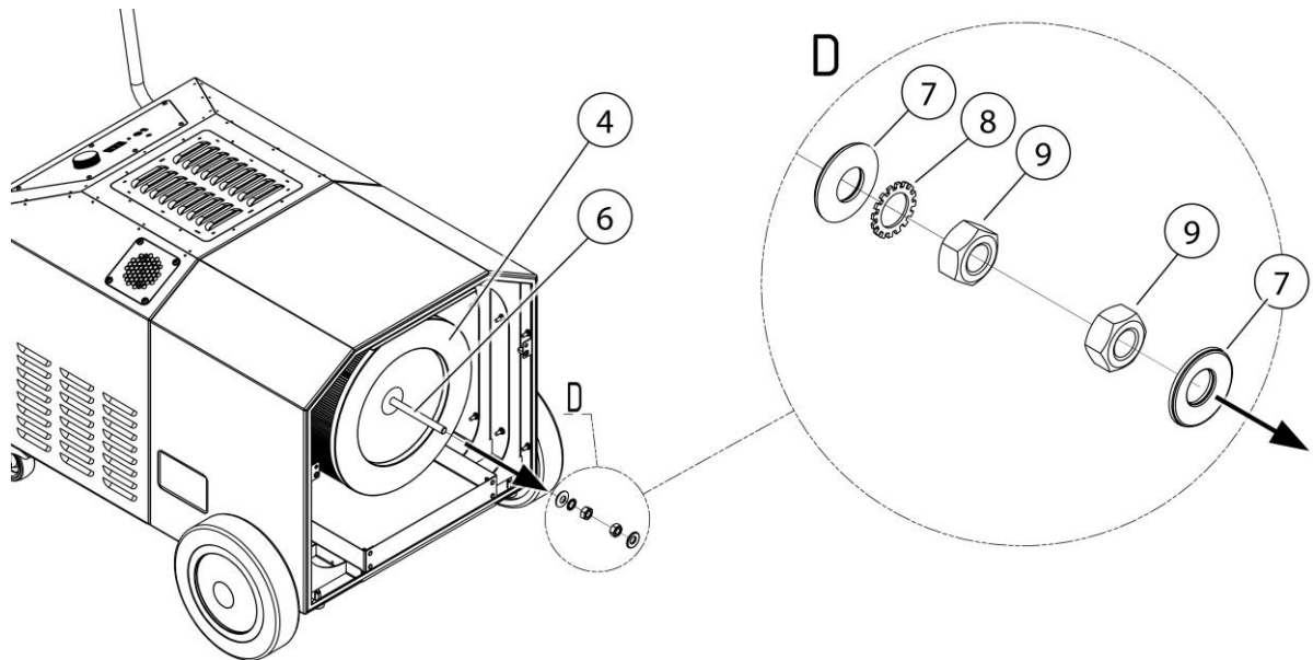
Abb. 10: Hauptfilter demontieren
