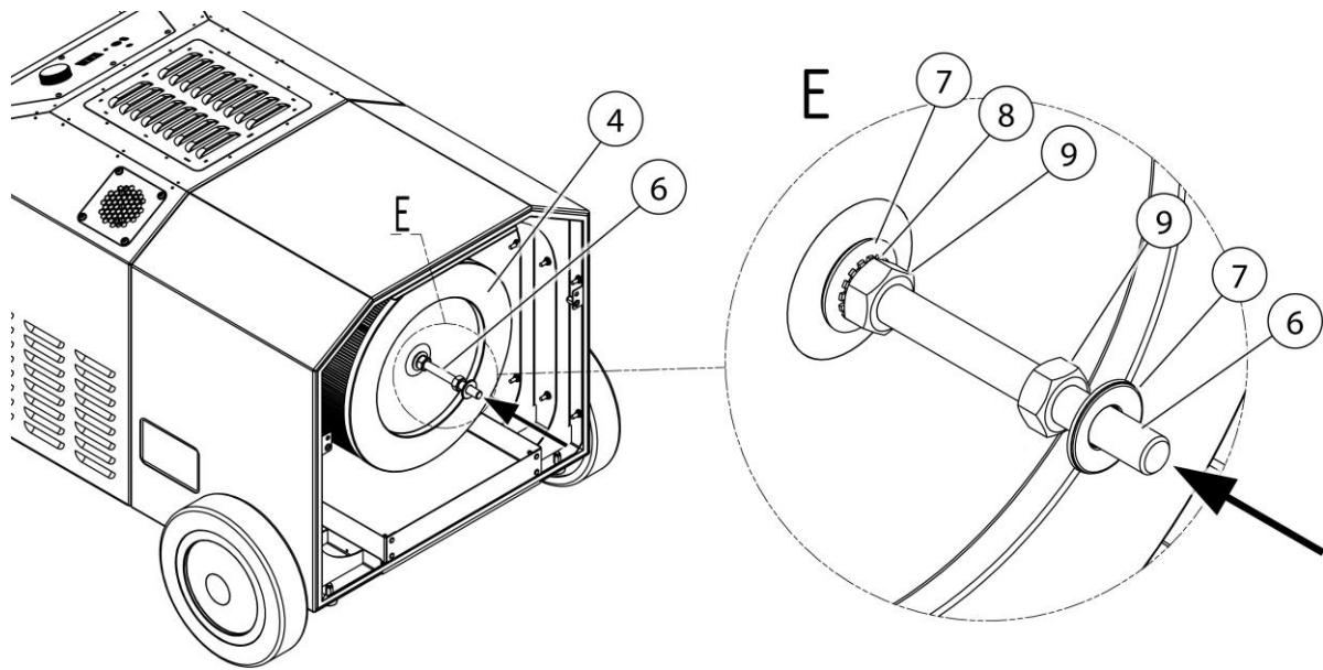
Abb. 13: Hauptfilter fixieren
