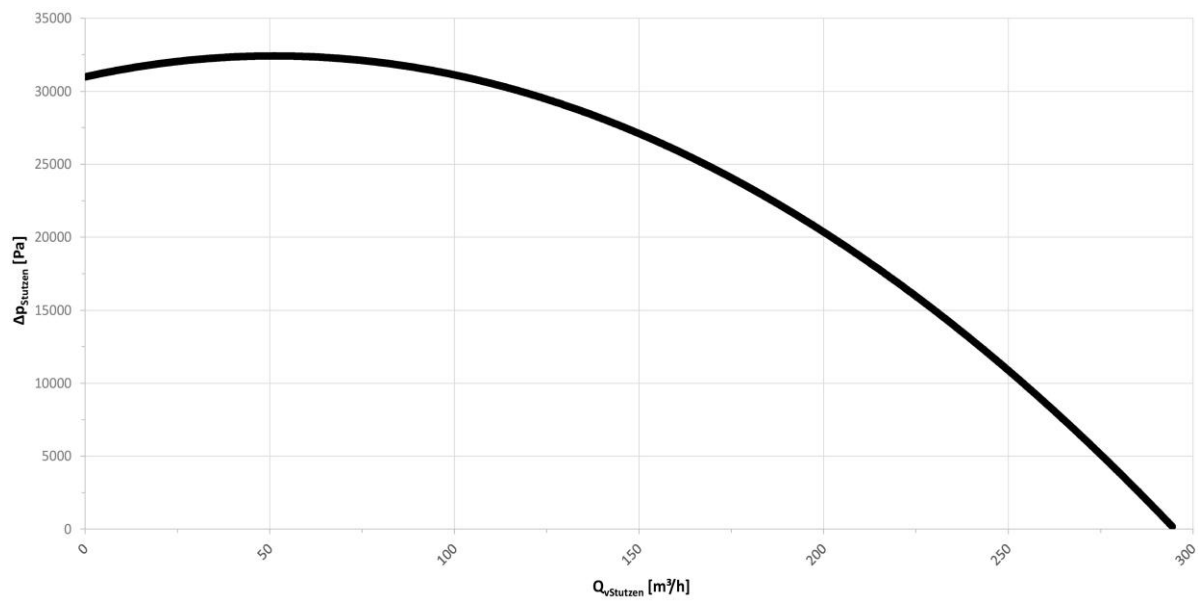
Abb. 16: Kennlinie
